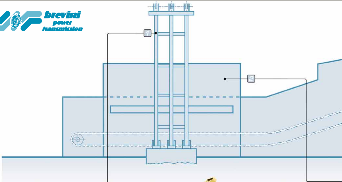
1 DESCARREGADORES TIPO 'HYLLO' CANE UNLOADERS 'HYLLO' TYPE DESCARGADORES TIPO 'HYLLO'
