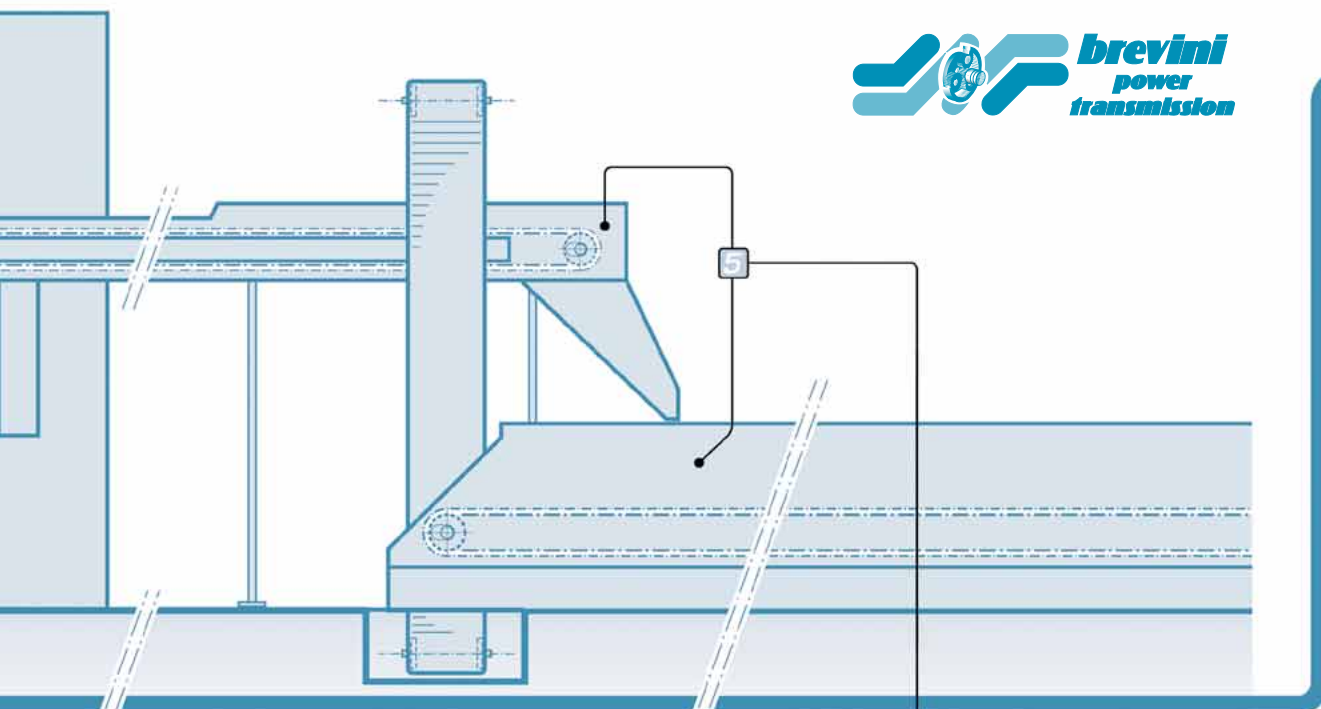
5 ESTEIRA DE DISTRIBUÇÃO DE BAGAÇO BAGASSE INFEEED CONVEYOR CONDUCTOR PARA DISTRIBUCIÓN DE BAGAZO
