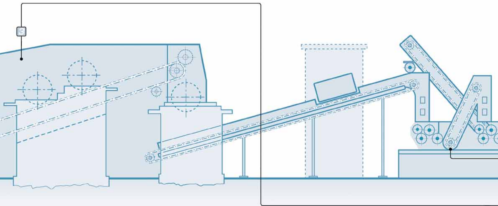
2 MESAS ALIMENTADORAS CANE FEEDERS AND WASHING TABLES MESAS DE ALIMENTACIÓN Y LAVADO
